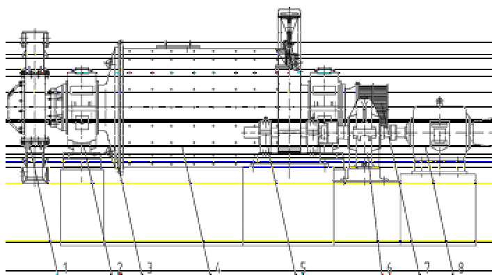
1. 联合给料器 2. 轴承箱 3. 进料部 4. 筒体部 5. 传动部 6. 减速机 7. 自料器 8. 电动机
